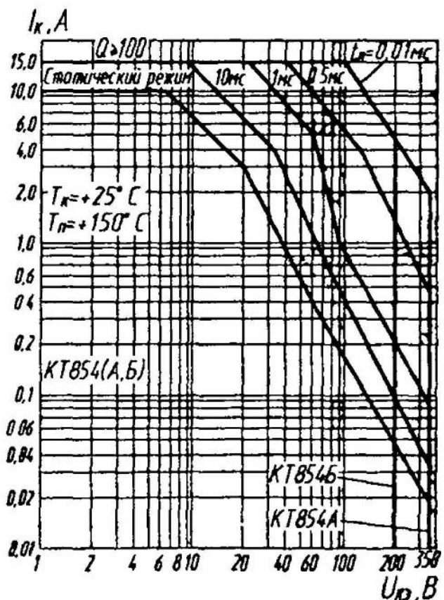
Области максимальных режимов
