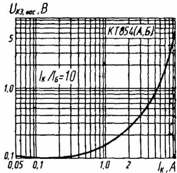
Зависимость напряжения насыщения коллектор—эмиттер от тока коллектора
