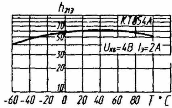
Зависимость статического коэффициента передачи тока от температуры
