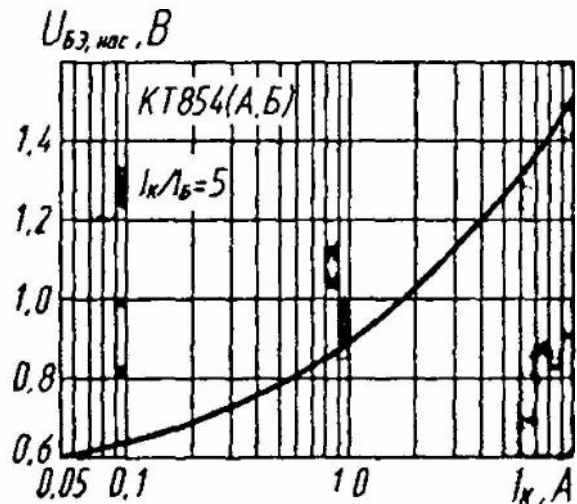
Зависимость напряжения насыщения база—эмиттер от тока коллектора
