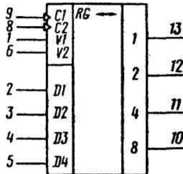
Условное графическое обозначение К155ИР1, КМ155ИР1
